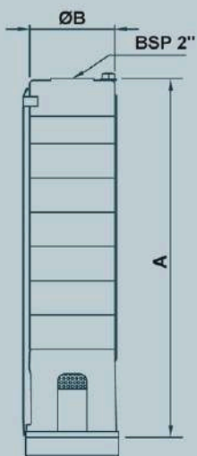
AM8/73 est monté dans un manchon / adaptateur en option
