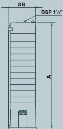
AM5/85 est monté dans un manchon / adaptateur en option
